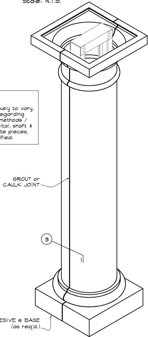
2 ASSEMBLED COLUMN Scale: N.T.S.
