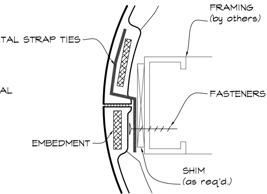
3 JOINT DETAIL Scale: N.T.S.
